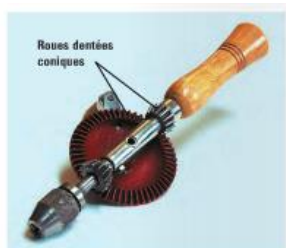
Figure 34 b Le système d'engrenage d'une chignole (perceuse à manivelle).
