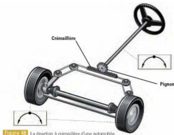
Figure 48 La direction à crémaillère d'une automobile.
