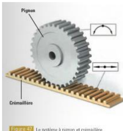
Figure 47 Le système à pignon et crémaillère.
